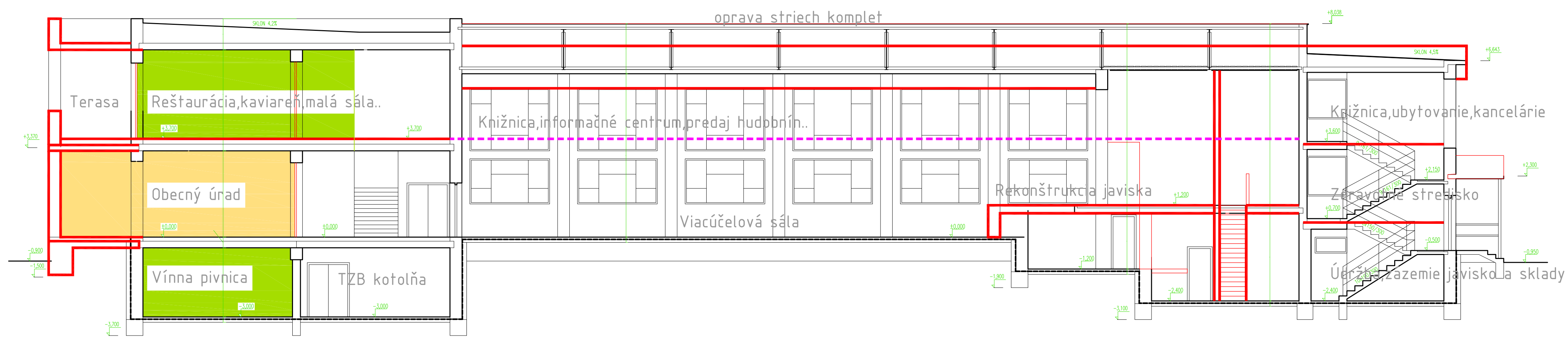
REZ POZDĚLNÝ M1:100
